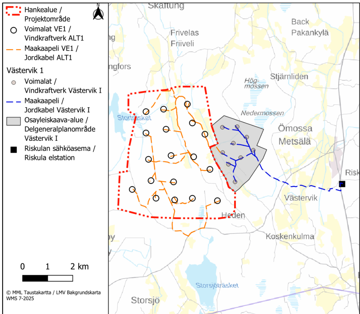
Bild 4. Jordkablar i Västervik II vindkraftsprojekt i projektalternativ ALT1.
