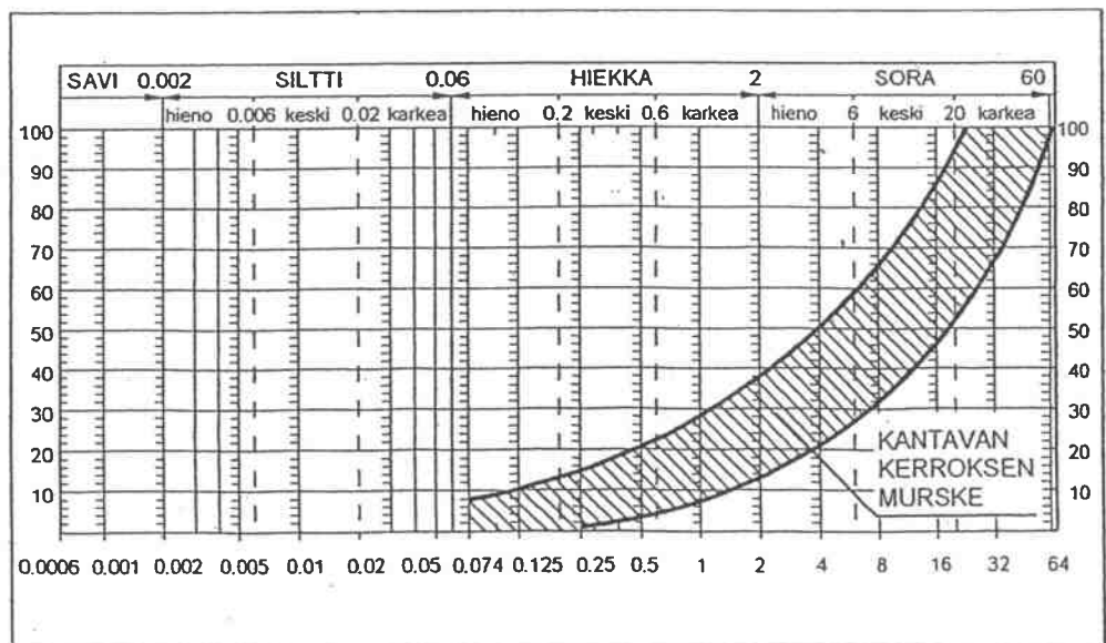
Kuva 26211: Kantavan kerroksen rakeisuuden ohjealue
