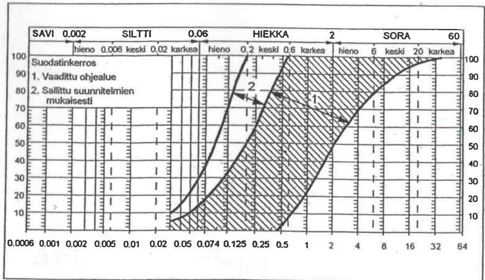
Kuva 26111: Suodatinkerroksen rakeisuuden ohjealue
