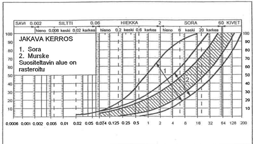
Kuva 26121: Jakavan kerroksen rakeisuuden ohjealue
