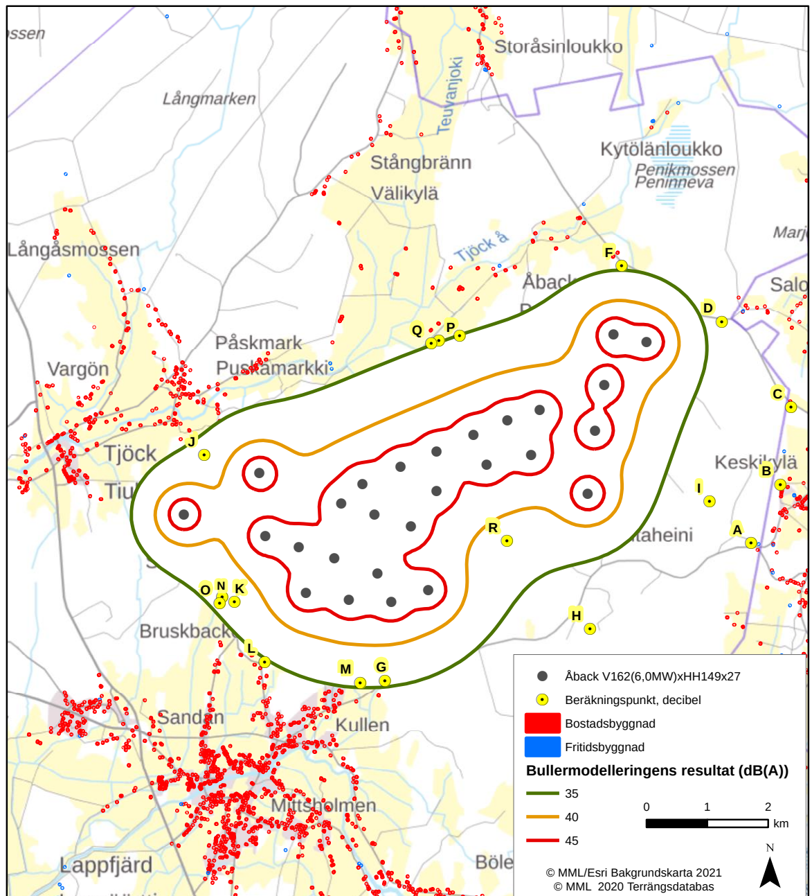
Bild 28. Bullermodelleringens resultat för Åback vindkraftsprojekt
