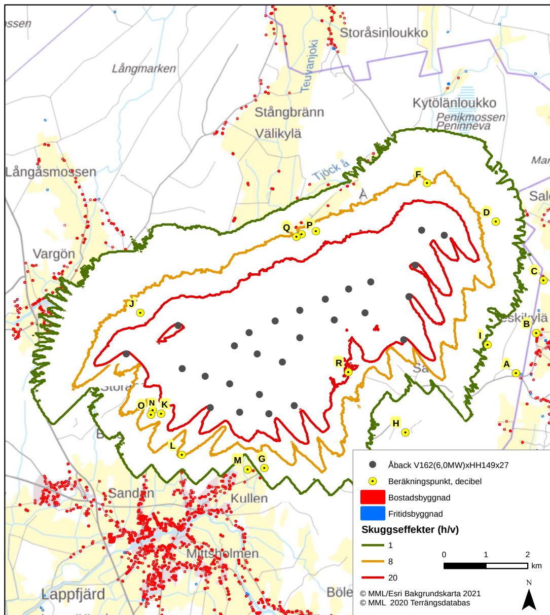
Bild 29. Skuggeffekter som orsakas av vindkraftverk utan inverkan från träden.
