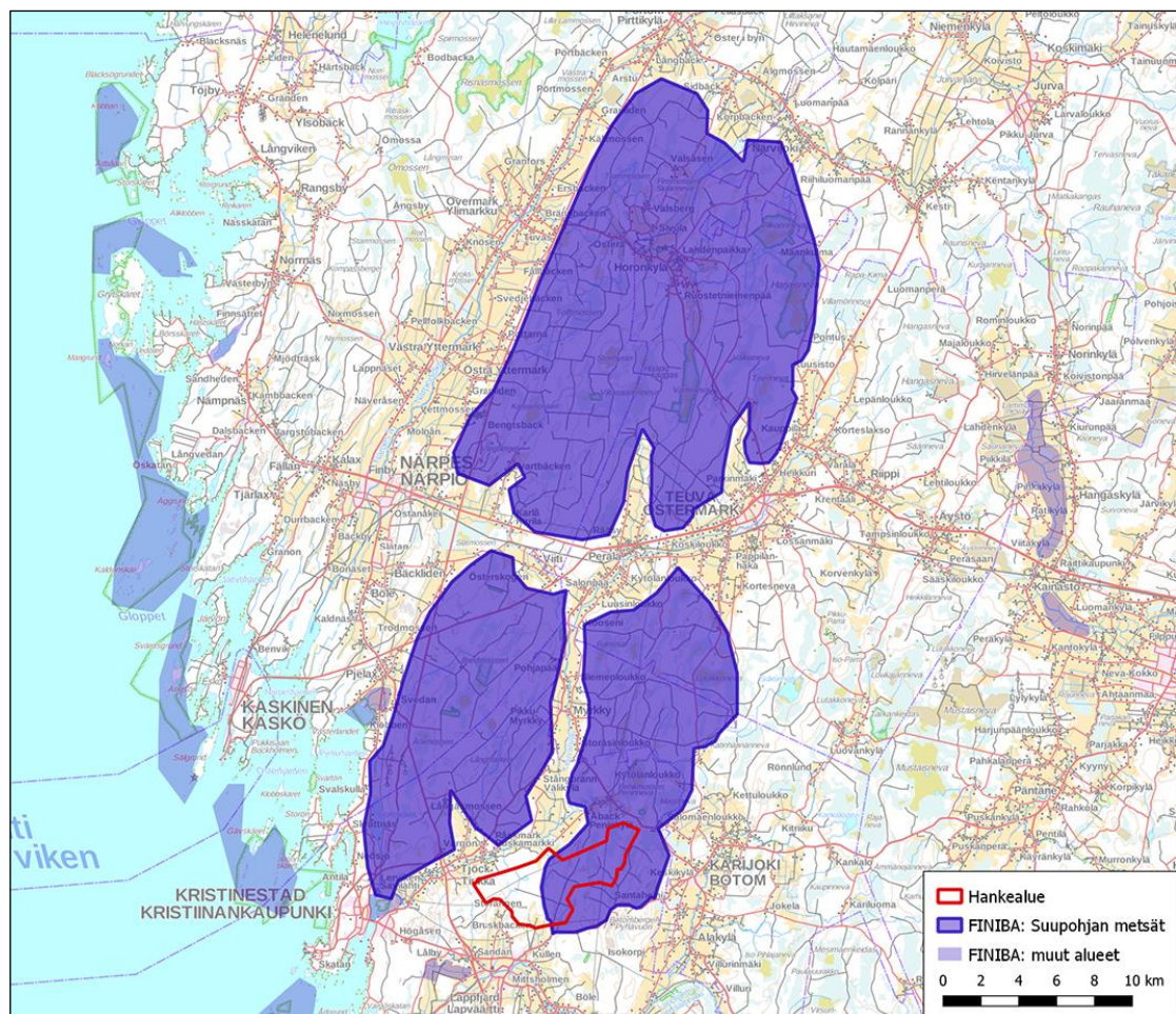
Bild 23. Placeringen av den planerade vindkraftsparken i Åre i förhållande till FINIBA-området Sydösterbottens skogar.
